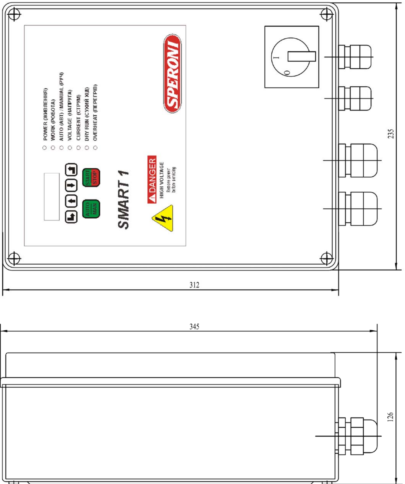
Рисунок А.1 – Общий вид устройства SMART-1
